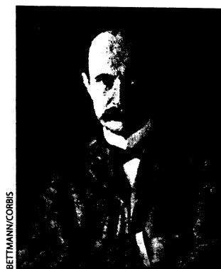
MAX PLANCK (1858–1947)
